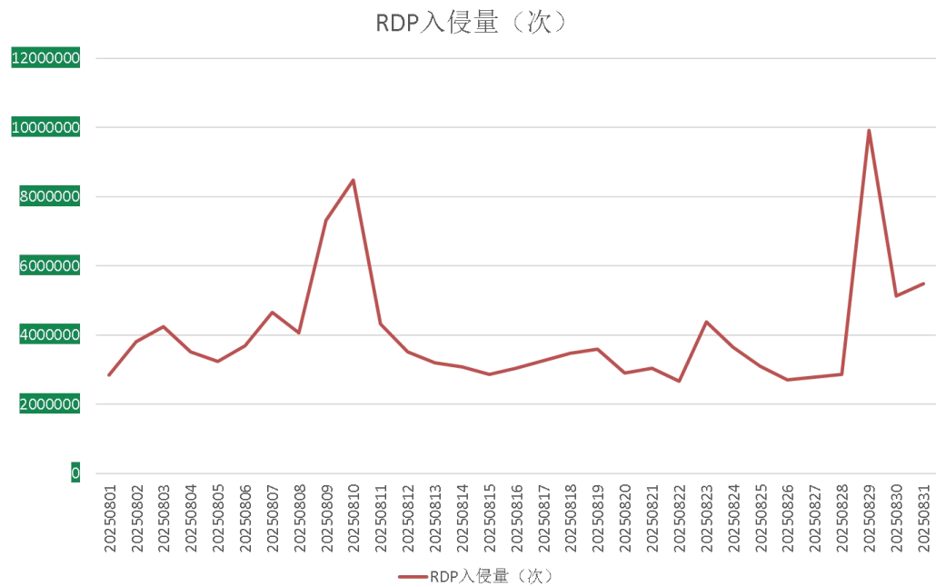
图 7. 2025 年 8 月监控到的 RDP 入侵量
