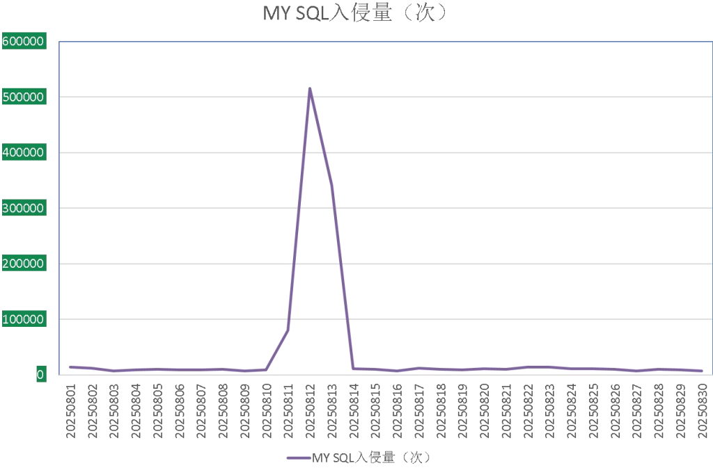
图 9. 2025 年 8 月监控到的 MYSQL 入侵量
