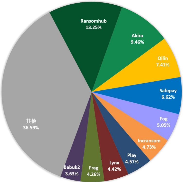
图 4. 2025 年 3 月通过数据泄露获利的勒索软件家族占比
