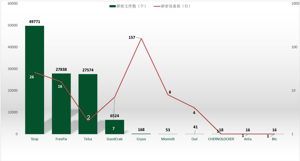
图 11. 2025 年 3 月解密大师解密文件数及设备数排名
