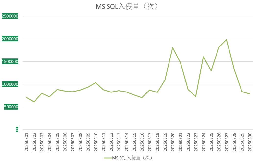
图 8. 2025 年 3 月监控到的 MS SQL 入侵量
