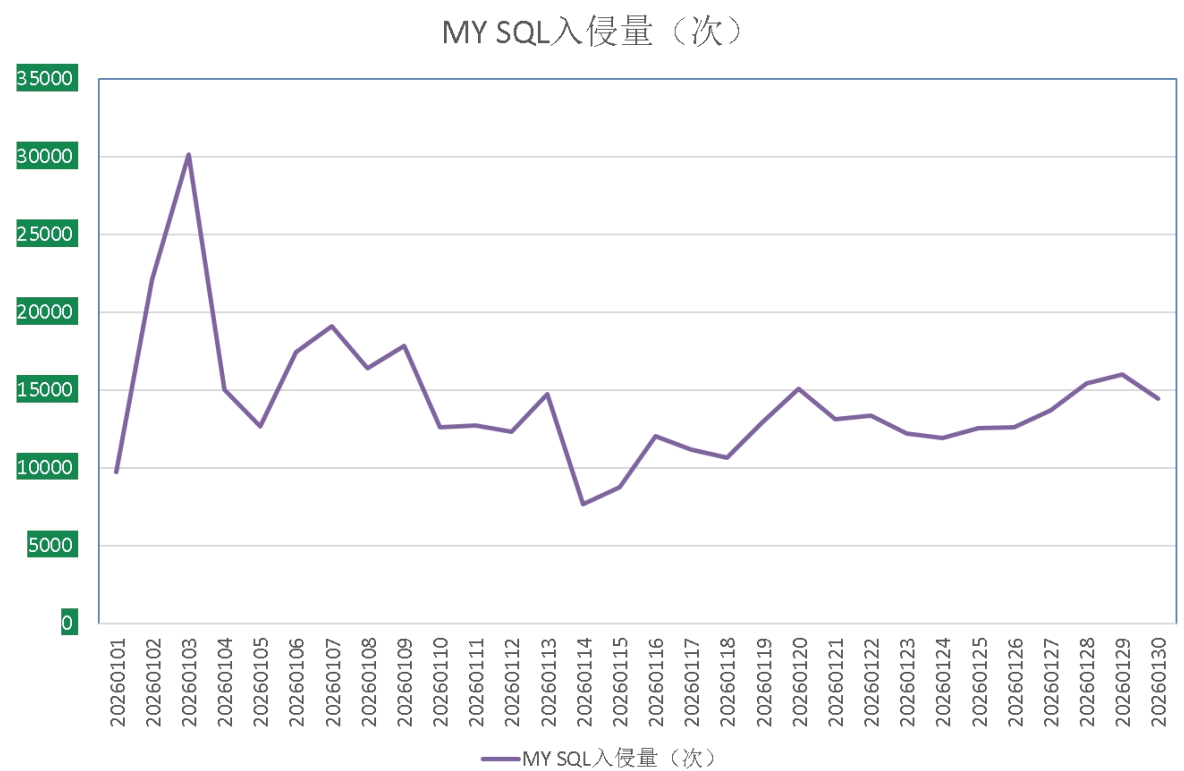
图 13. 2026 年 1 月监控到的 MYSQL 入侵量
