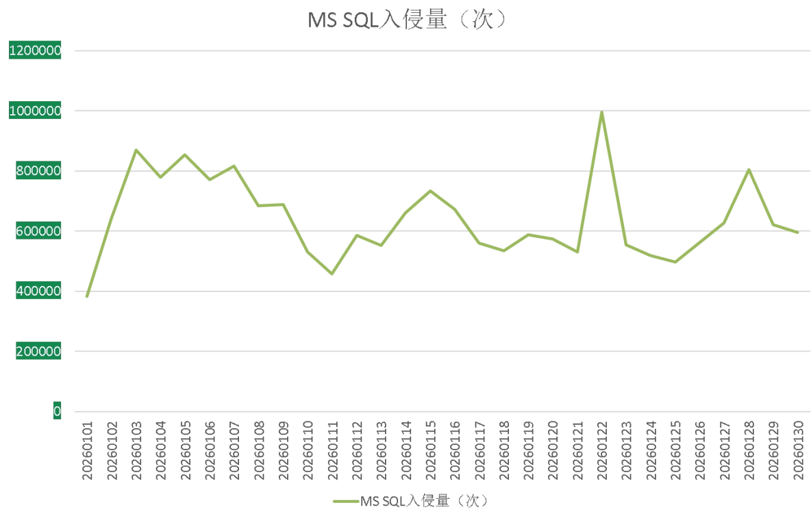
图 12. 2026 年 1 月监控到的 MS SQL 入侵量
